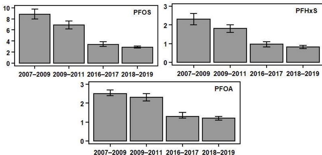
図 V-976 カナダ人口 CHMS で得られた人における血漿中 PFAS 濃度の経時変化 (Health Canada 2023) (参照 255)
