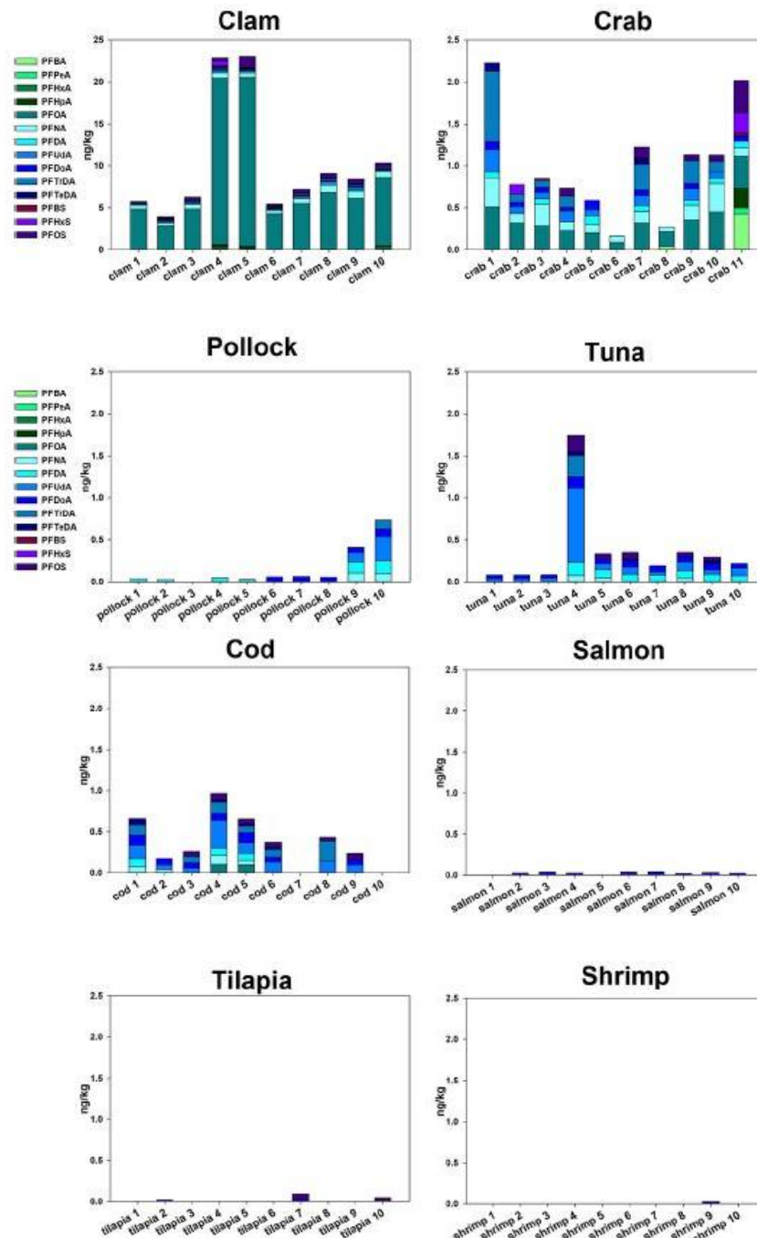
図 V-2 FDA の による 2021～2022 年魚介類調査サンプル中の PFAS 濃度（グラフ）
