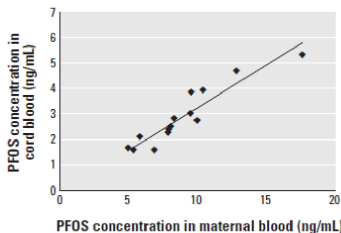
図 V-1198 妊婦の母体血清と臍帯血清の中 PFOS 濃度と臍帯血中 PFOS 濃度の相関
