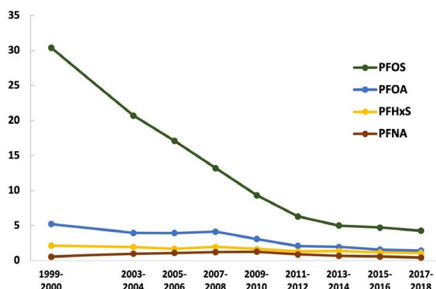
図 V-658 米国 NHANES で得られた人における最も一般的な PFAS の血中濃度の経時変化 (ATSDR 2023) (参照 254)
