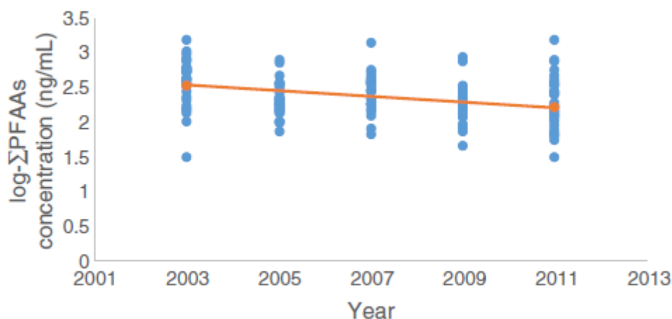
図 V-1209 母体血漿中 総 PFAS のパーフルオロアルキル酸濃度の経年変化の時間的 傾向
