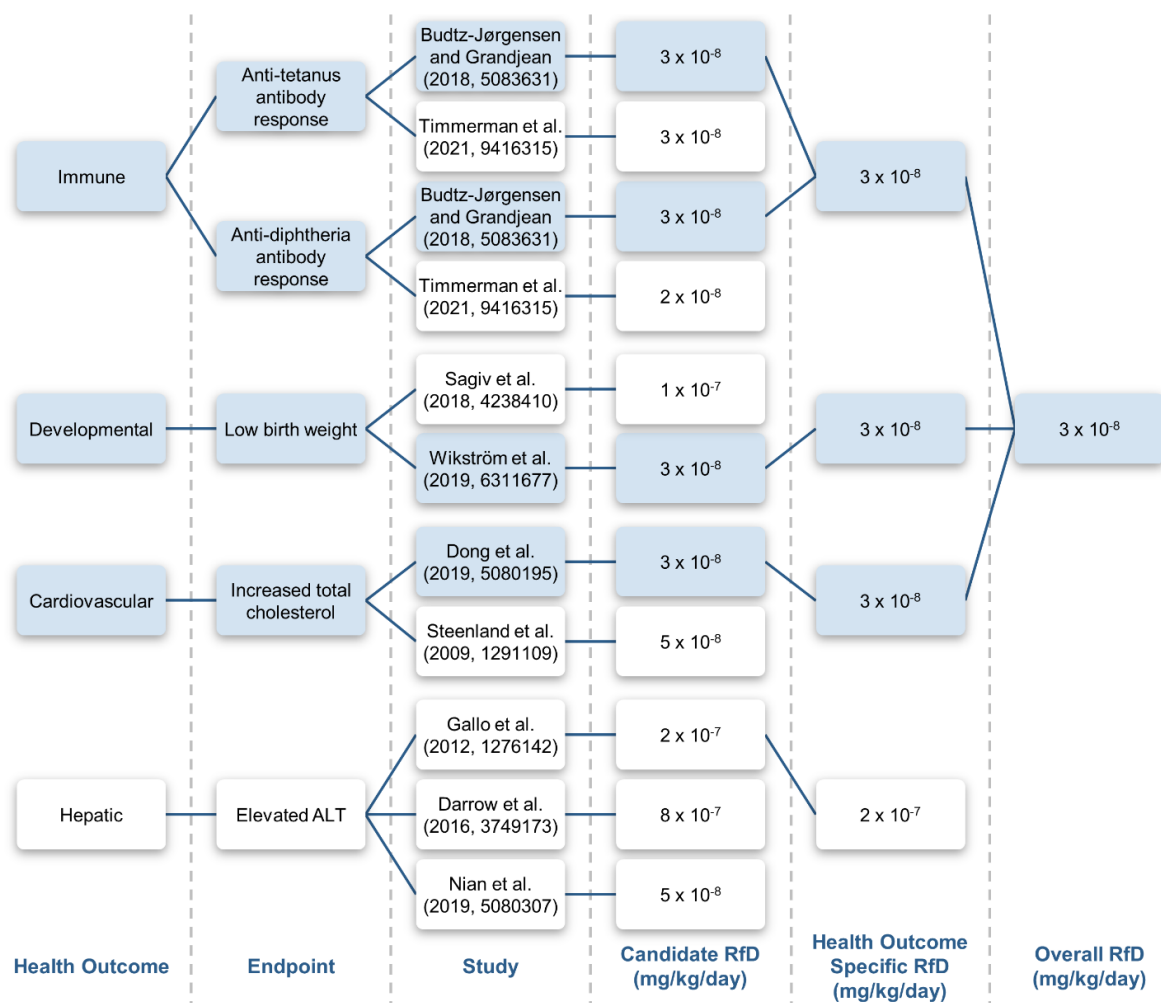
図Ⅸ-Ⅶ-2PFOA の RfD 設定スキーム（EPA 2023 の Figure-4-4. Schematic depicting selection of the overall RfD for PFOA を転載）
