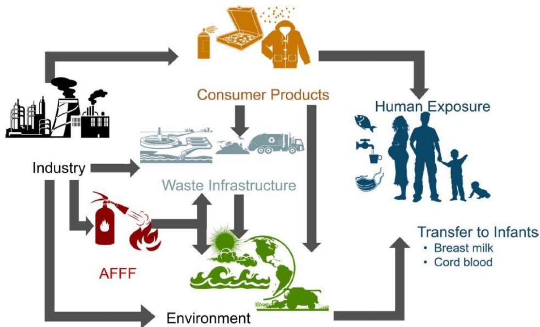
図 V-1 ヒトにおける職業性ばく露以外の環境外におけるからの様々なヒト集団のPFAS ばく露経路の概要 (Sunderland et al. 2019) (参照 227)
